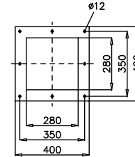
Ansicht X
